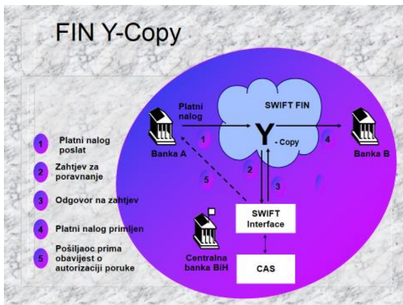
Слика 2. Принцип рада Свифт Y-Цопу сервиса
