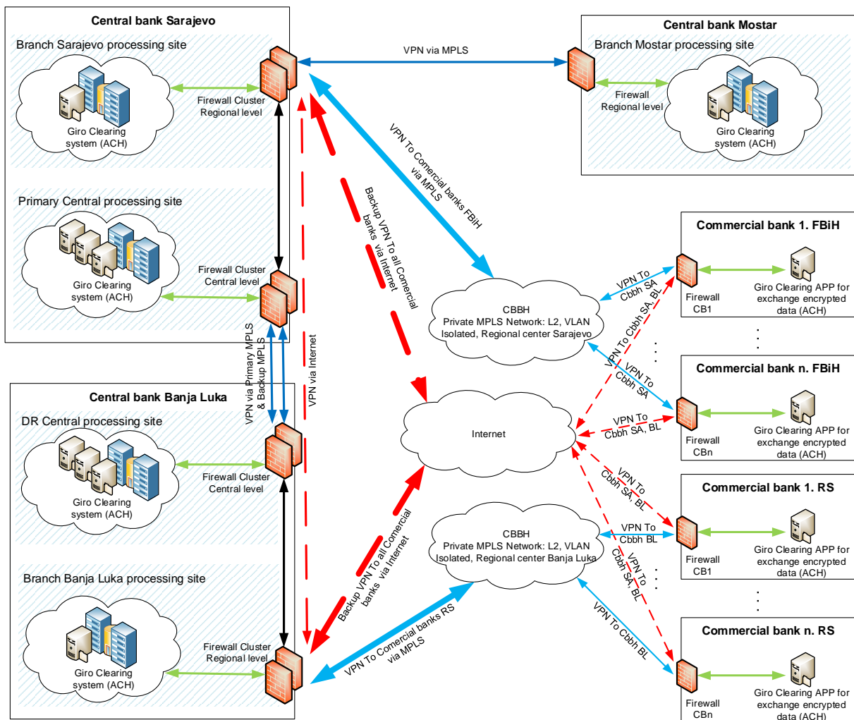
Слика 1. Глобална схема жироклиринг система
