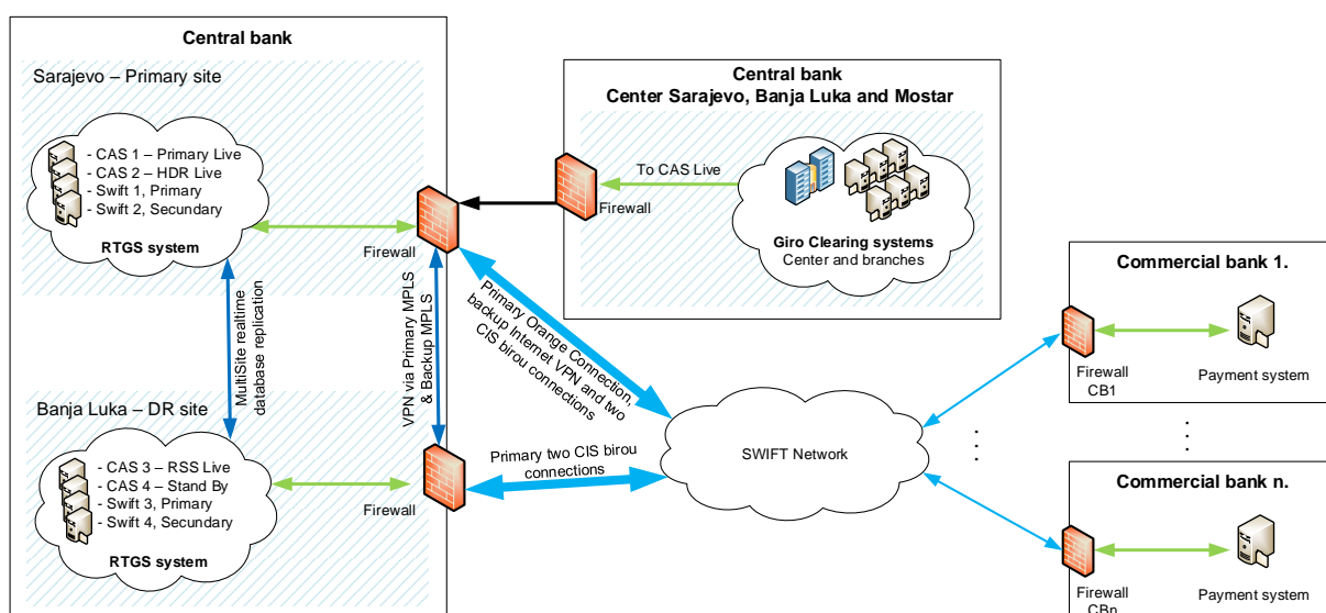
Слика 3. Глобална схема RTGS система
